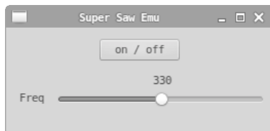
Figure 3. Interface graphique.
