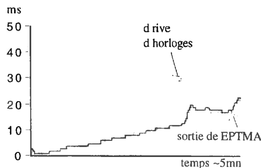
Figure 7: sortie de EPTMA comparé à PTMA
