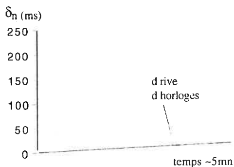
Figure 3: mesure de la variation de la latence pendant 5 mn
