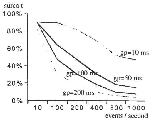
Figure 2: surcoût des protocoles sous-jacents en fonction de la période de groupage et de la fréquence des événements.
