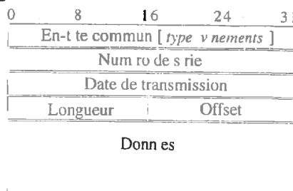
Figure 9: format des paquets d'événements
